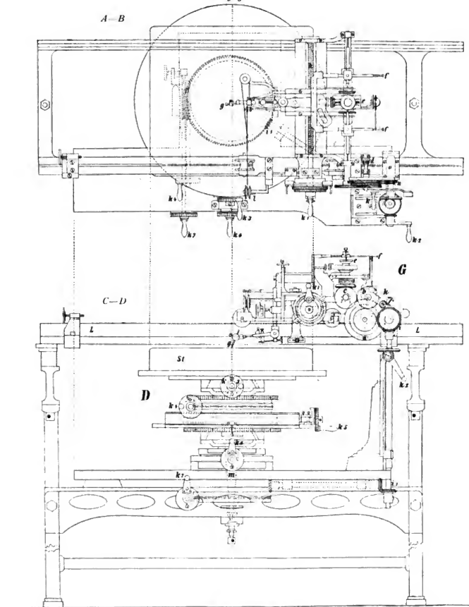
Grosse Guillochirmaschine.
