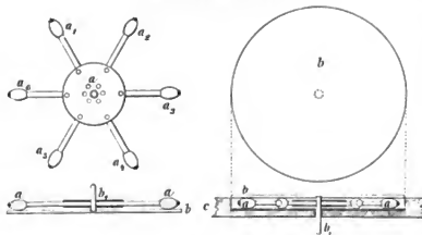
Detailzeichnung zu Fig. 23. \frac{1}{10} der Originalgröße.
