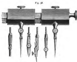
Stangenzeirkel mit Einsatzstücken.
