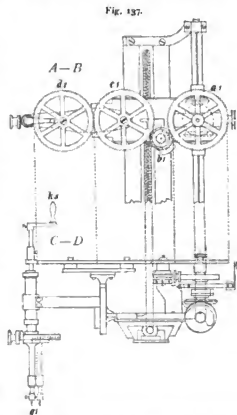
Fig. 137. Schleifenlinien - Apparat zur grossen Guillochirmaschine.
