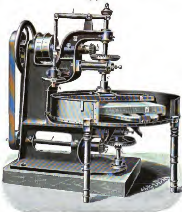
Universal-Rundsleifmaschine von G. Eckhardt in Leipzig-Rendnitz.
