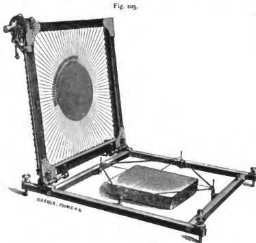
Reduktionsapparat „Diagonal“ mit unterlegtem Stein und Fadenkreuzung.
