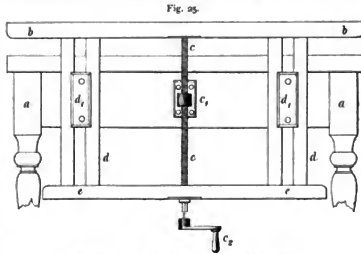
Detailzeichnung zu Fig. 23, \frac{1}{10} der Originalgröße.
