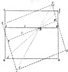
Schema des Mailänder oder Fünftangen-Pantographen.
