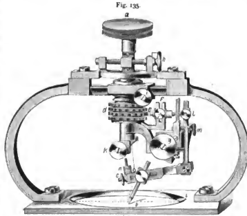
Kleine Guillochmaschine.
