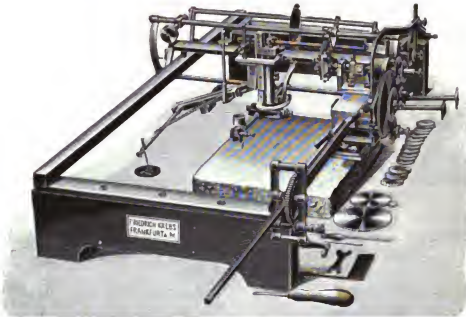
Wellen- und Reliefmaschine.
