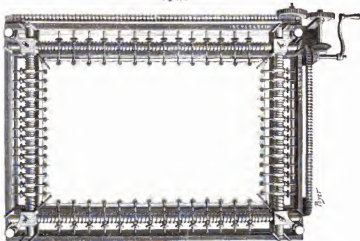
Reduktionsapparat mit Kettenantrieb.
