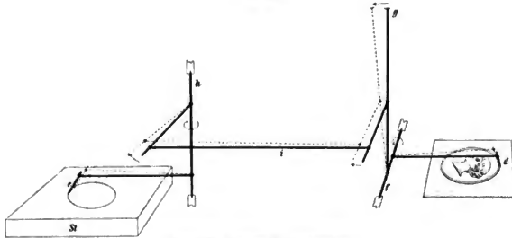
Prinzipielle Darstellung der Reliefmachine.
