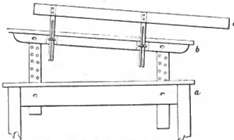
Detailzeichnung zu Fig. 20. \frac{1}{10} der Originalgröße.
