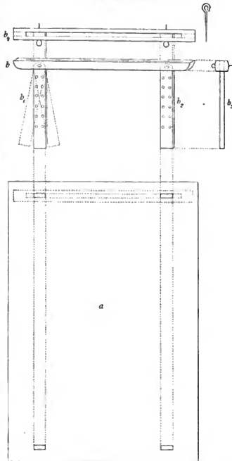
Detailzeichnung zu Fig. 20, \frac{1}{10} der Originalgrösse.
