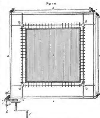
Reduktionsapparat mit Stirnräderantrieb.
