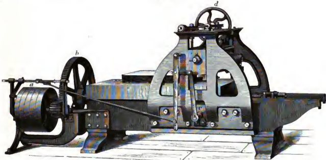
Steinhobelmaschine der Schnellpressenfabrik Hugo Koch in Leipzig.
