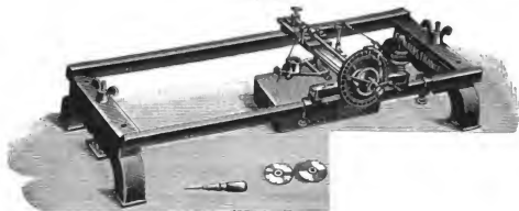
Einfache Linirmaschine.
