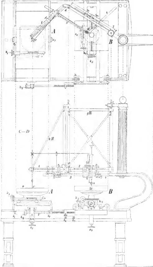
Der grosse Gravirpantograph.
