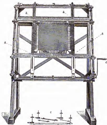
Pieper's Original-Präzisions-Pantograph für Buntdruck.
